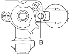
Thermostatgeregelter Gashahn B Einstellschraube für minimale Wärmebelastung
