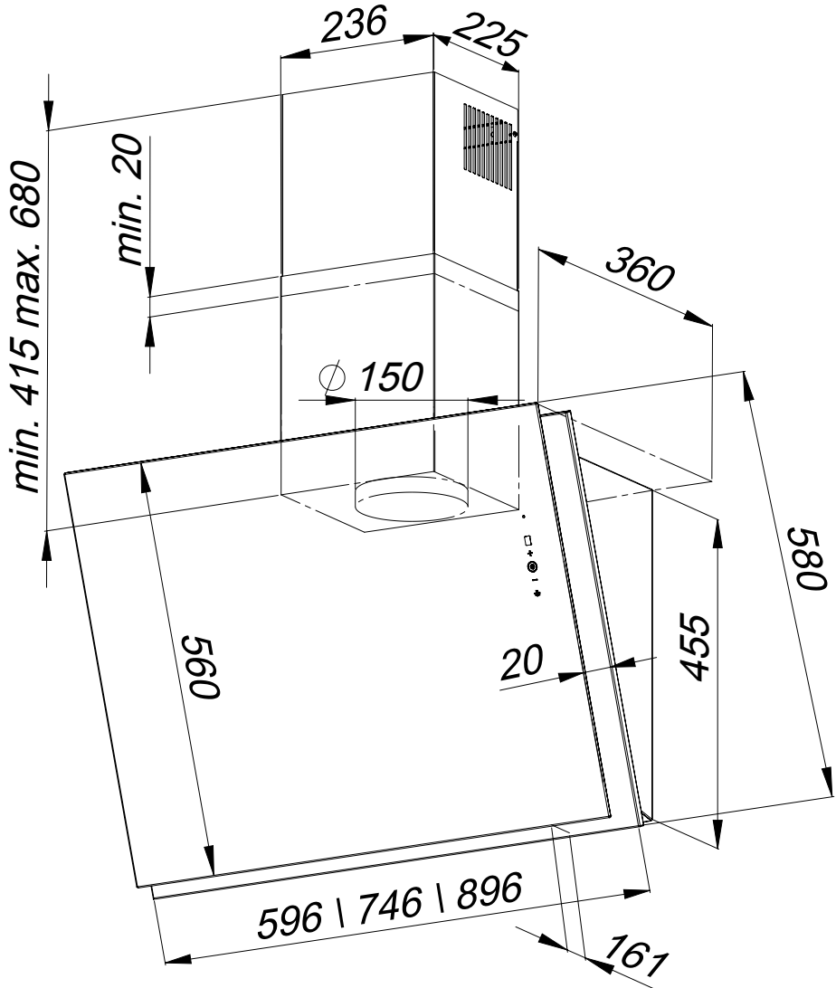
Abb. 18 Abmessungen Modelle „Davara“
